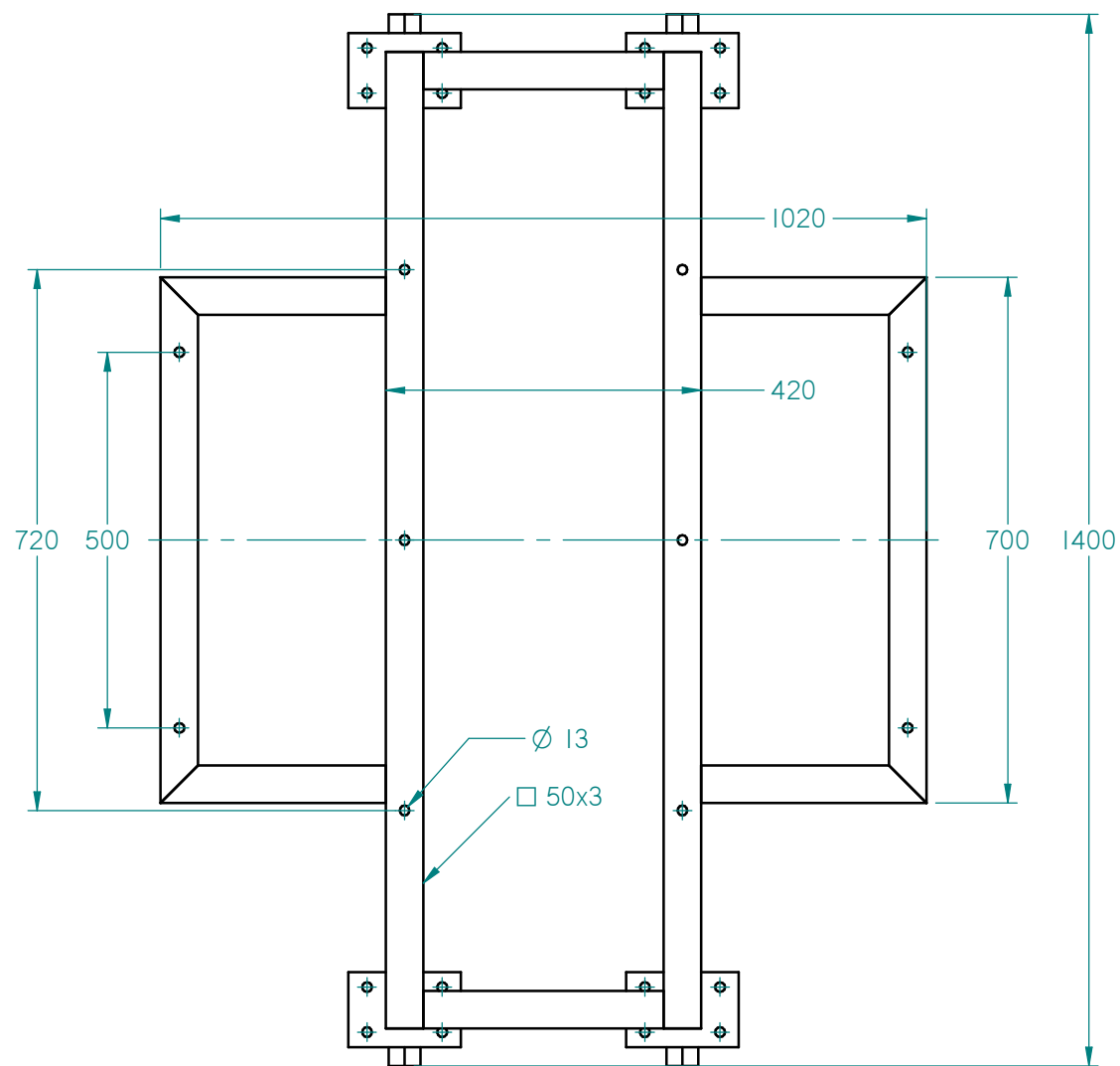
PS-D1-1300-3 Držák příhrady hmotnost : 38 kg
